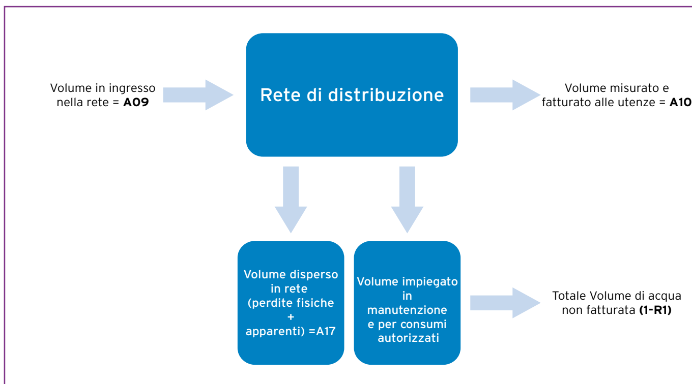
Fig. 1 - Schema dei Volumi nella rete di Distribuzione
