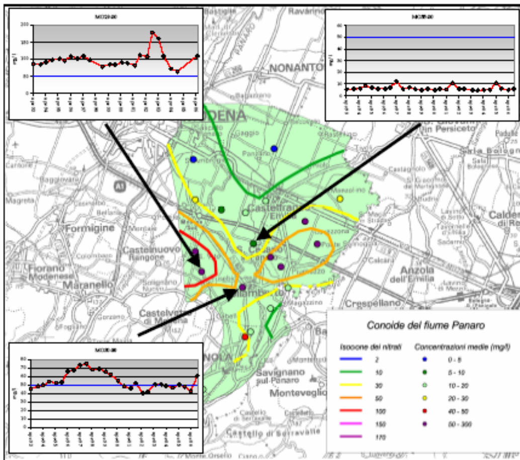
Fig. 4.16 Distribuzione areale e puntuale delle concentrazioni di nitrati – anno 2006
