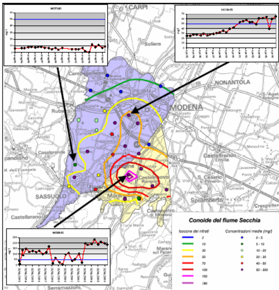
Fig. 4.19 Distribuzione areale e puntuale delle concentrazioni di nitrati – anno 2006
