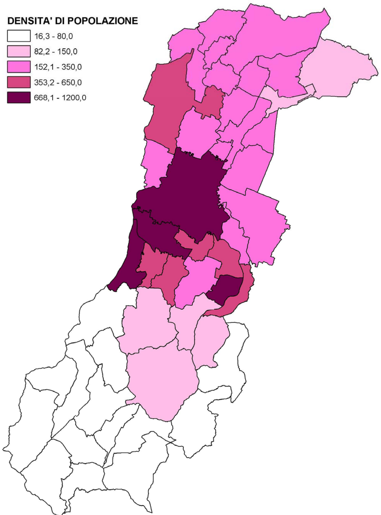
Fig. 3.2 Densità demografica (abitante/kmq) nella Provincia di Modena
